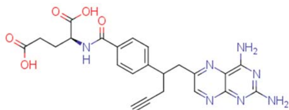
146464-95-1
