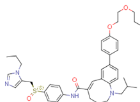
497223-28-6
