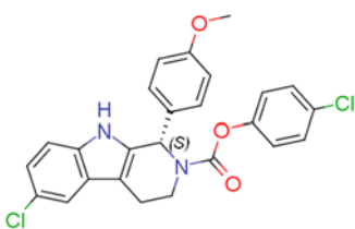
1256565-36-2
