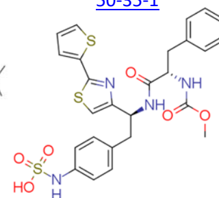
1008510-37-9
