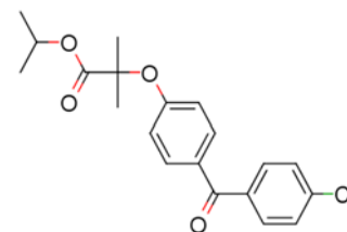
49562-28-9
