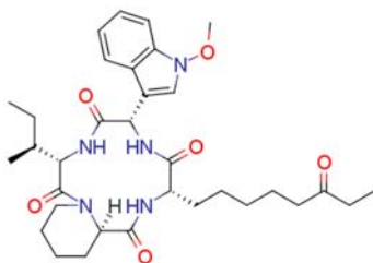
183506-66-3
