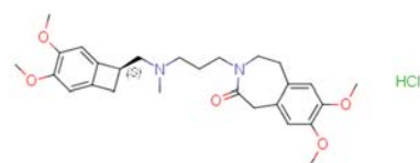
148849-67-6
