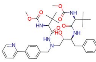
198904-31-3
