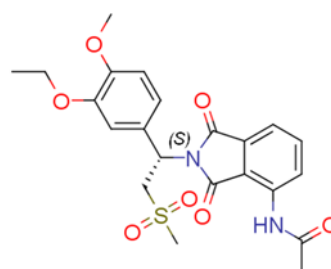
608141-41-9
