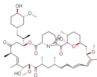
53123-88-9
