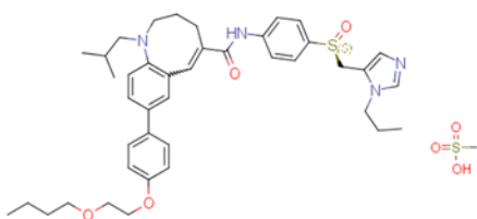
497223-25-3
