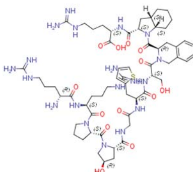
130308-48-4
