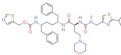
544-31-0
