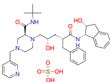
157810-81-6
