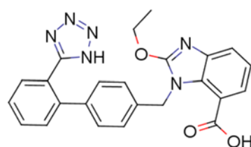
139481-59-7
