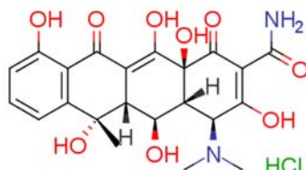
2058-46-0
