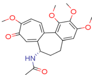
64-86-8
