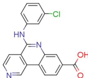
1009820-21-6
